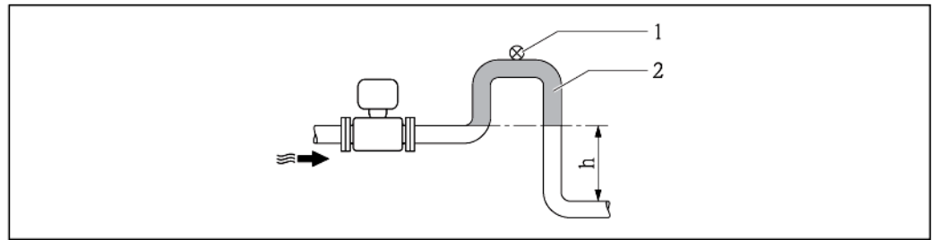
4 Монтаж в спускной трубе
