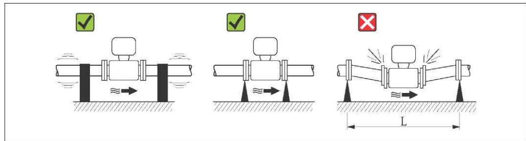
5 Меры по предотвращению вибрации прибора ( L > 10\text{ м} )
