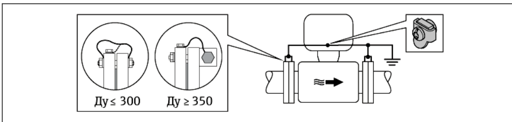
10 Контур заземления с использованием клеммы заземления и фланцев трубы
