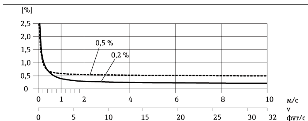
■ 16 Максимальная погрешность измерения в % ИЗМ
