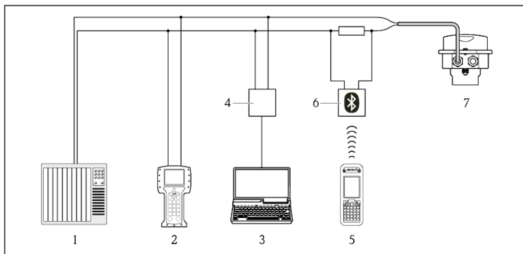
18 Варианты дистанционного управления по протоколу HART
