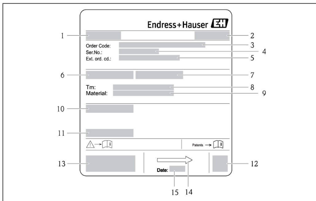
3 Образец заводской таблички сенсора
