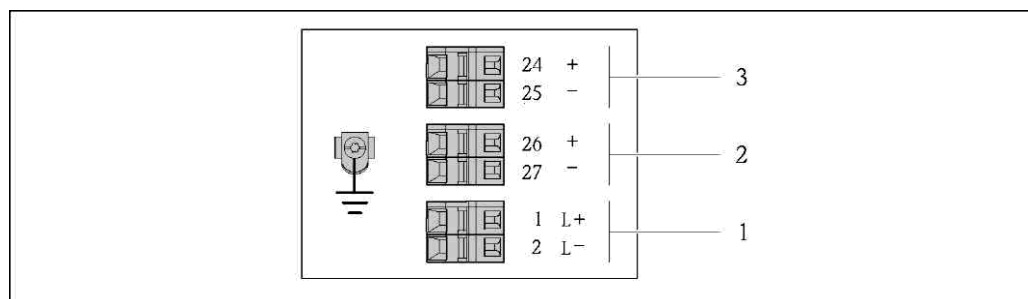
6 Назначение контактов: 4...20 мА HART с импульсным/частотным/релейным выходом
