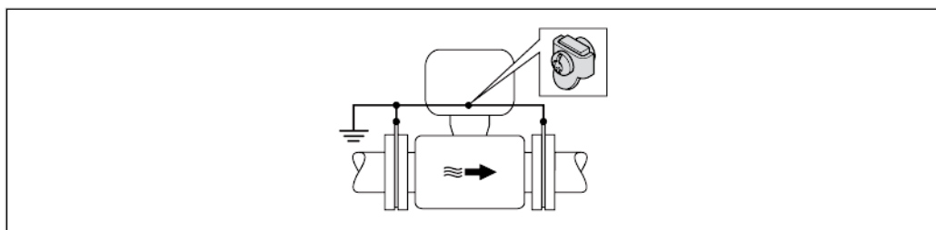
11 Контур заземления, реализованный с помощью клеммы заземления и заземляющих дисков
