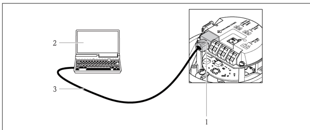
19 Подключение для кода заказа "Выход"1, опция В: 4...20 мА HART, импульсный/частотный/релейный выход
