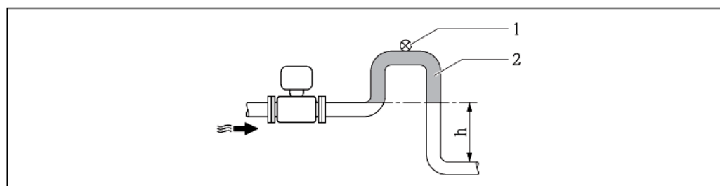
10 Монтаж в спускной трубе
