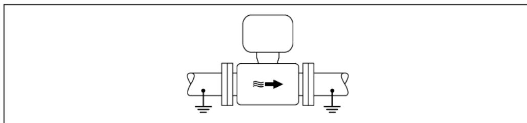
6 Контур заземления, реализованный с использованием измерительной трубы
