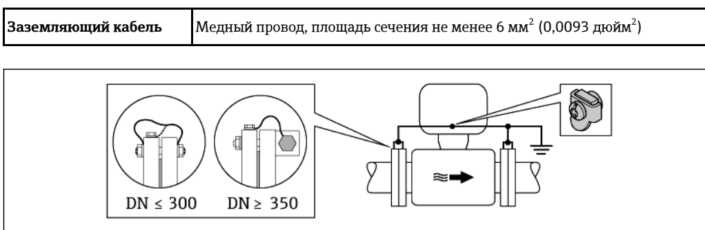
7 Контур заземления, реализованный с использованием клеммы заземления и фланцев трубы
