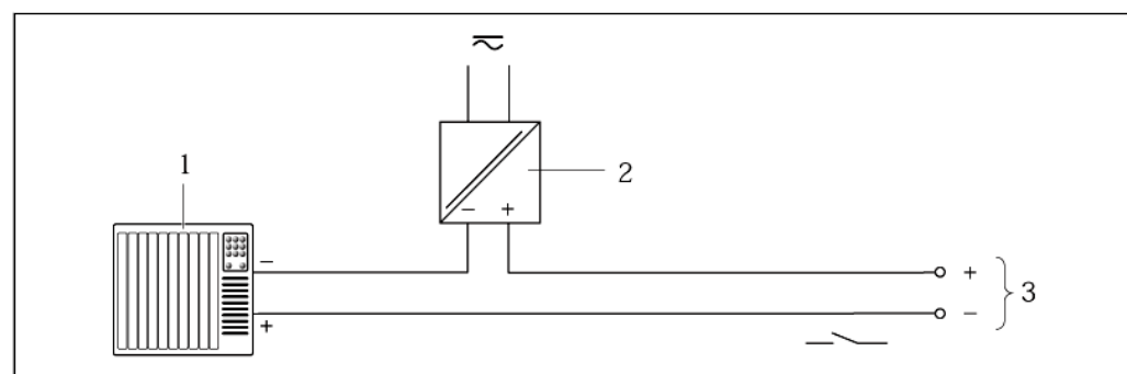
3 Пример подключения релейного выхода (пассивного)
