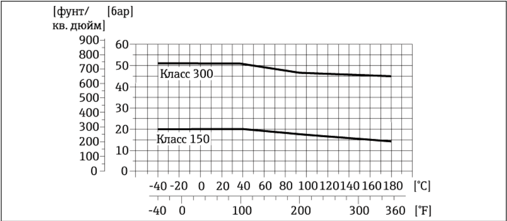
13 Материал присоединения к процессу, углеродистая сталь, A105
