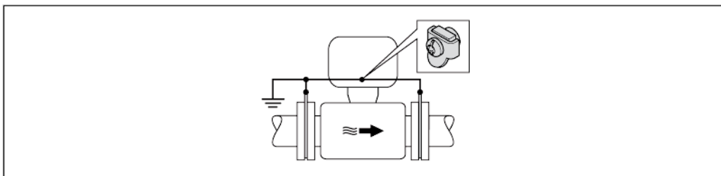
8 Контур заземления, реализованный с помощью клеммы заземления и заземляющих дисков
