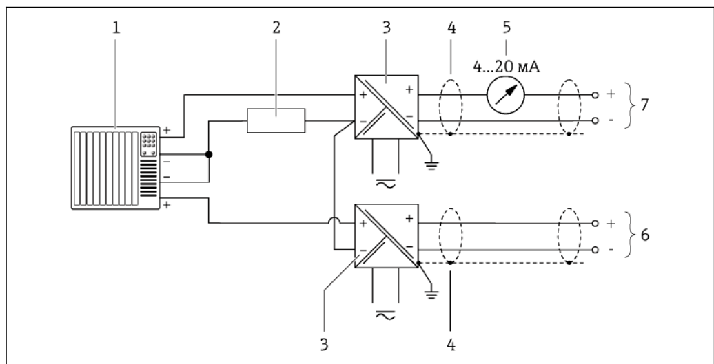
5 Пример подключения для входа HART с общим минусом
