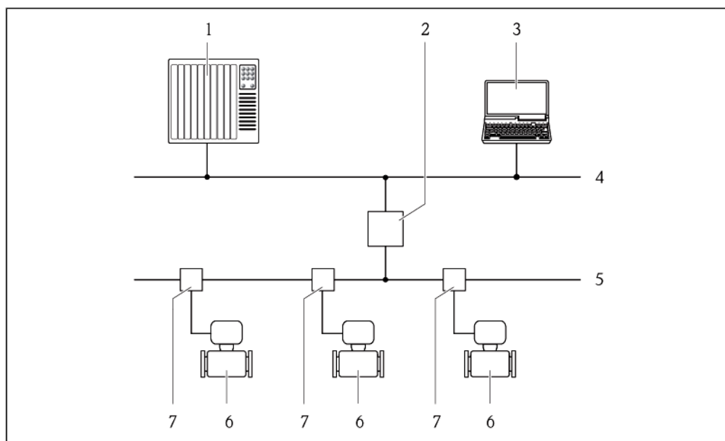
20 Варианты дистанционного управления по сети PROFIBUS PA
