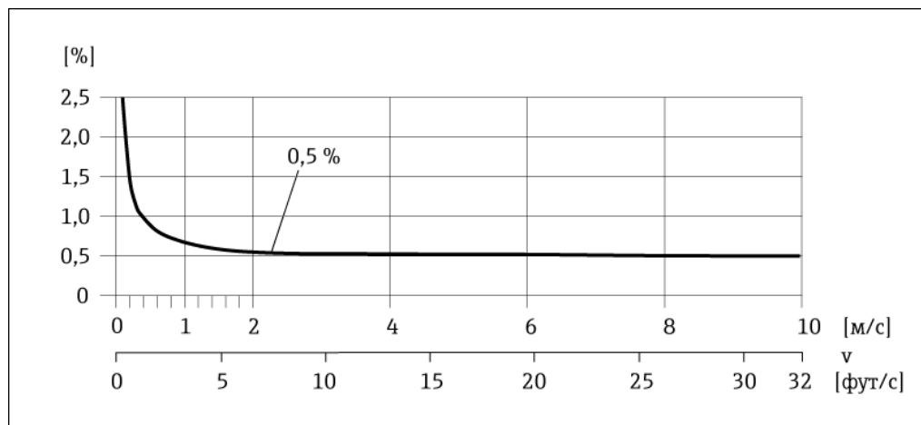
9 Максимальная погрешность измерения в % ИЗМ
