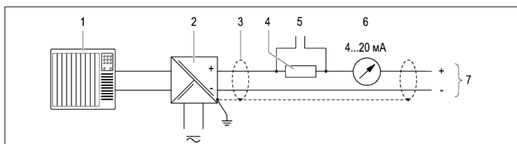
1 Пример подключения для пассивного токового выхода 4...20 мА HART
