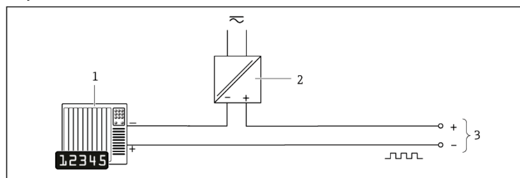
2 Пример подключения импульсного/частотного выхода (пассивного)
