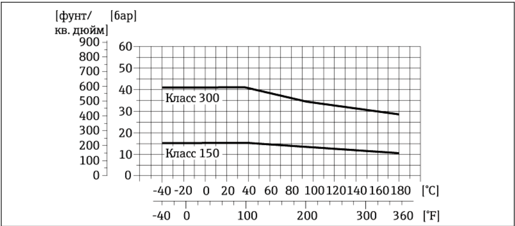
14 Материал присоединения к процессу: нержавеющая сталь, F316L
